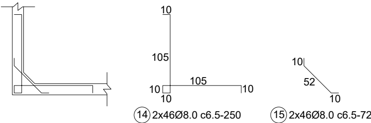
Detalhe 02: Ligação Fundo – Parede escala 1/50
