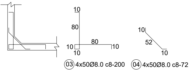
Detalhe 01: Ligação Parede = Parede escala 1/50
