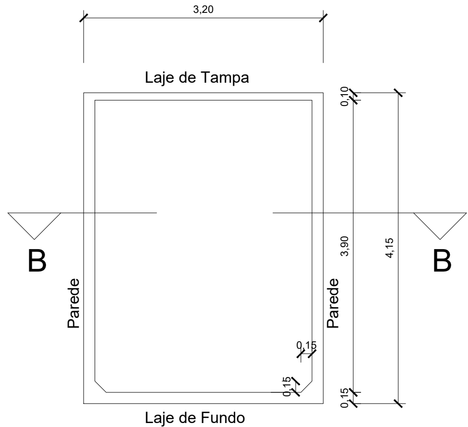
Corte Vertical AA escala 1/50
