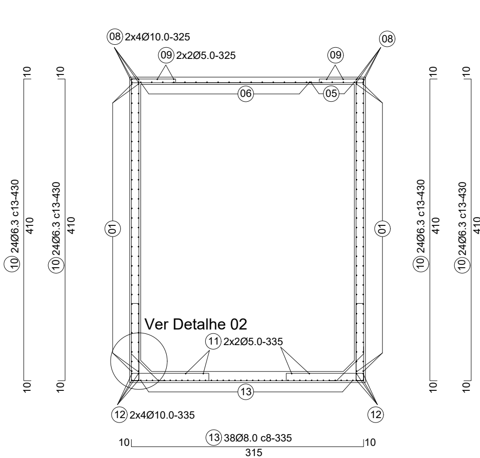
Armação do Corte Vertical AA escala 1/50
