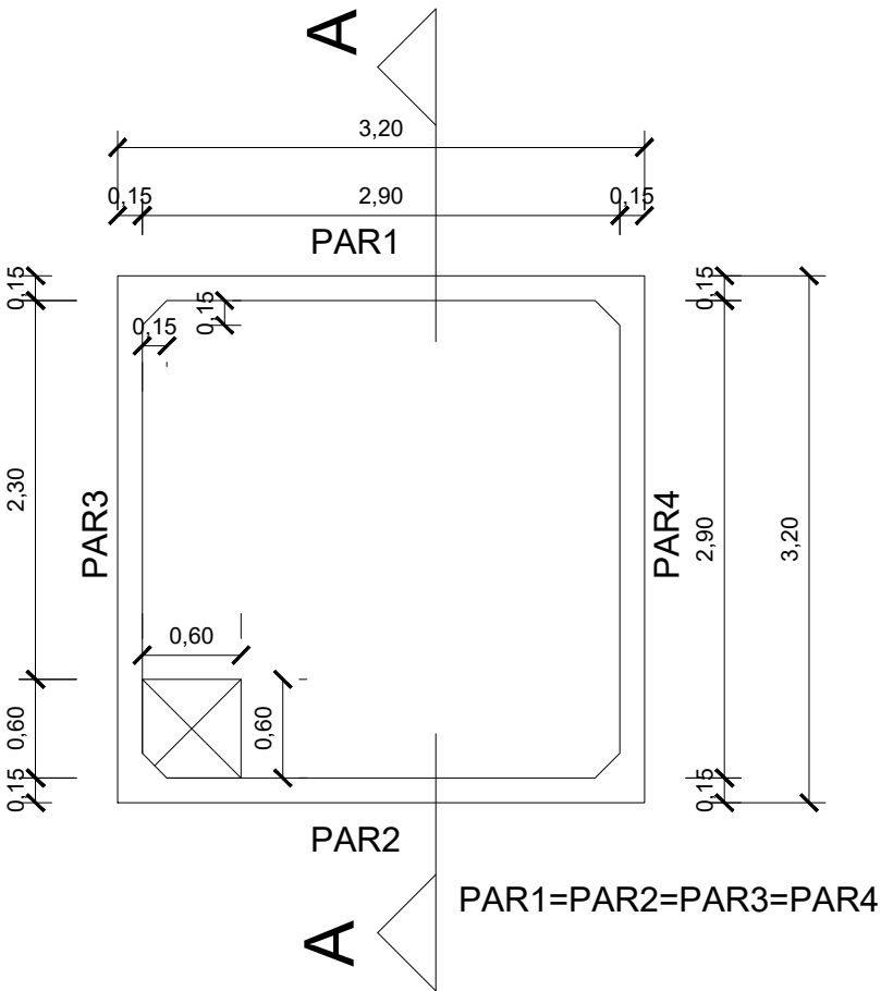
Forma Reservatório – Reservatório Superior escala 1/50
