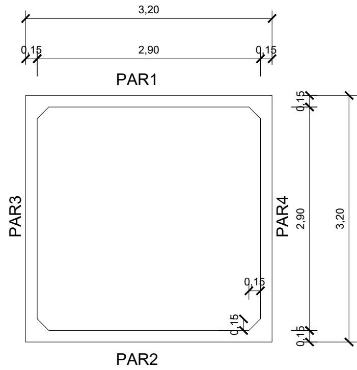
Corte Horizontal BB escala 1/50
