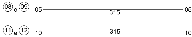
Detalhe das Armadura – 8,9,11 e 12 escala 1/50
