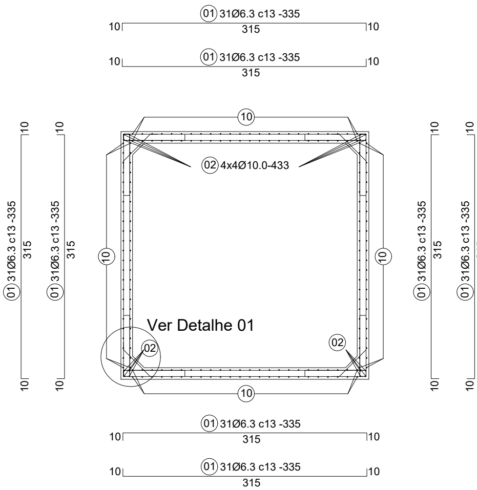
Armação do Corte Horizontal BB escala 1/50
